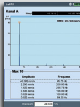
Värähtelyanalyysi auttaa tunnistamaan ja poistamaan koneviiat.
