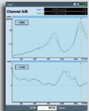
Yksi- tai kaksikanavainen alasajotesti joko RMS:nä, amplitudina tai vesiputouksena.
